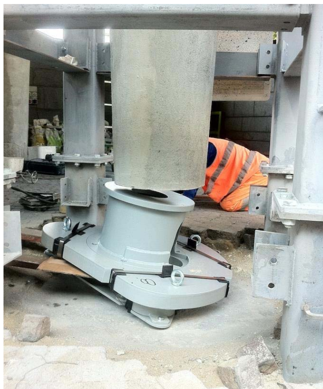
Figura 9. Inserimento dei "tripodi" sotto i pilastri, preventivamente tagliati alla base.
