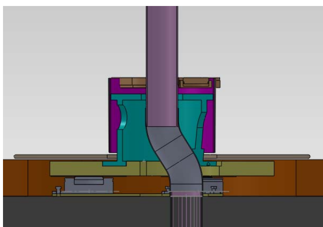
Figura 8. Il "tripode": vista e sezione. Si noti il particolare del condotto di scarico dotato di gomito deformabile.
